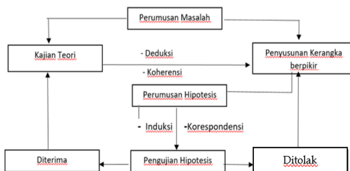
Gambar 2. Desain penelitian
